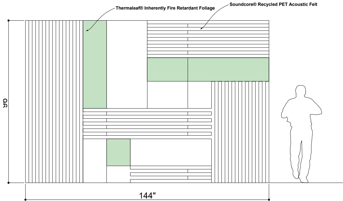
② ELEVATION 2
