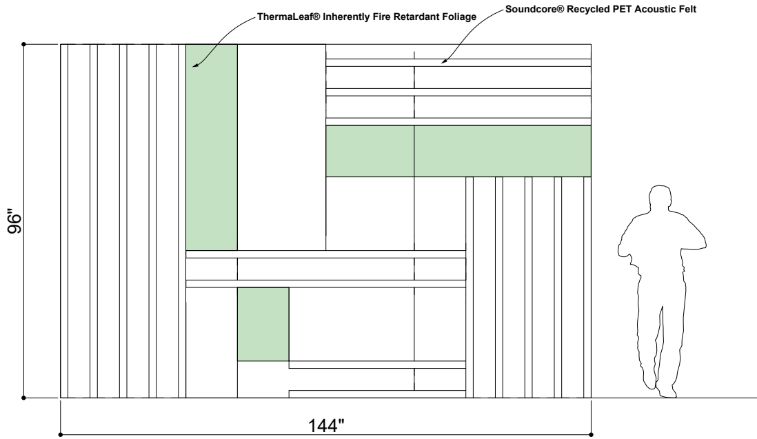
① ELEVATION 1
